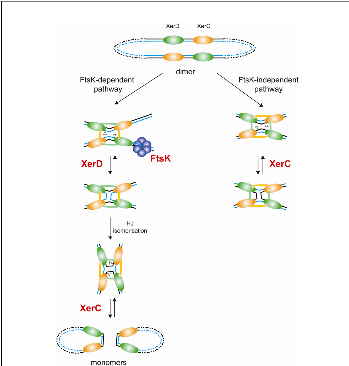
Figure 28. Voie de recombinaison Xer à dif dépendante et indépendante de FtsK En l'absence de FtsK, le complexe synaptique adopte une conformation où XerC est plus favorisée pour cliver. La jonction de Holliday formée est reconvertit en substrat par XerC. FtsK utilise l'énergie d'hydrolyse de l'ATP pour activer XerD dans le complexe synaptique. Il y a alors formation d'une jonction de Holliday productive qui peut être résolue par XerC indépendamment de FtsK. XerC est représenté en gris clair et XerD en gris foncé. FtsK est représentée sous forme hexamérique. L'action de coupure de XerC et XerD est représentée par des triangles blancs et noirs respectivement.
