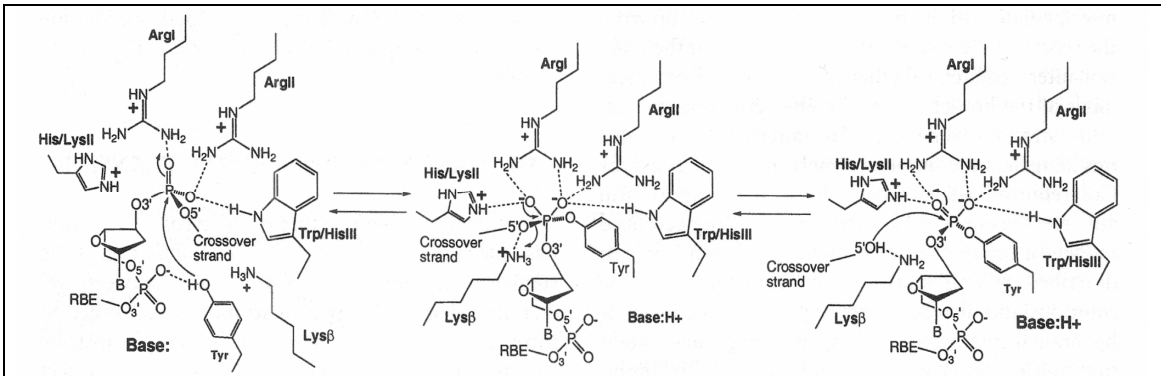
Figure 12. Mécanisme de coupure et de ligation des recombineses à tyrosine par réaction de transesterification (Van Duyne, 2002).
