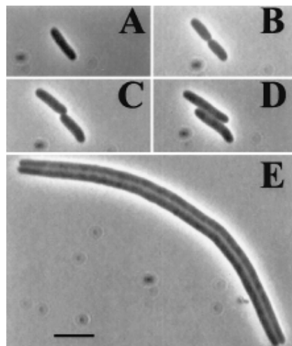
Figure 25. Formation de filaments jumeaux ('Twin filaments') formés par division et élongation de mutants de E. coli ne pouvant pas résoudre leurs dimères de chromosomes ( \Delta dif-hipA::cat , PK3946) (Hendricks et al. , 2000). Les cellules vivantes sont étalées sur une lame de microscope recouverte de milieu agar. Les photos sont prises à intervalles durant la croissance des cellules à 37°C. L'échelle indique 5 \mu m. (A) Cellule initiale (B) Après 15 min, (C) Après 30 min, (D) Après 45 min, (E) Après 120 min.
