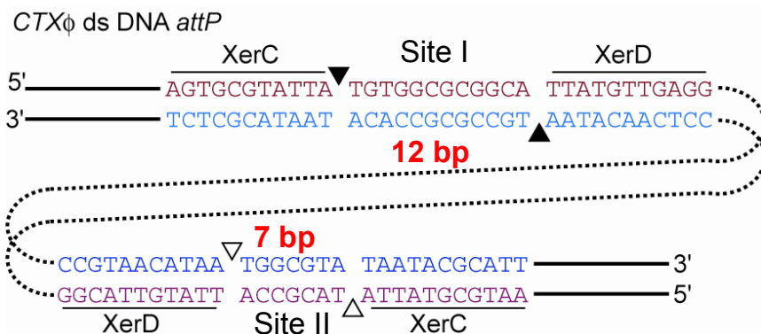
Figure 45. Représentation des sites I et II du site attP séparés par une séquence de 90pb dans la forme répliative double brin de CTXφ.
